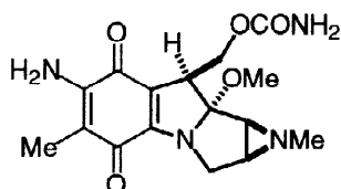
Mitomycin C
